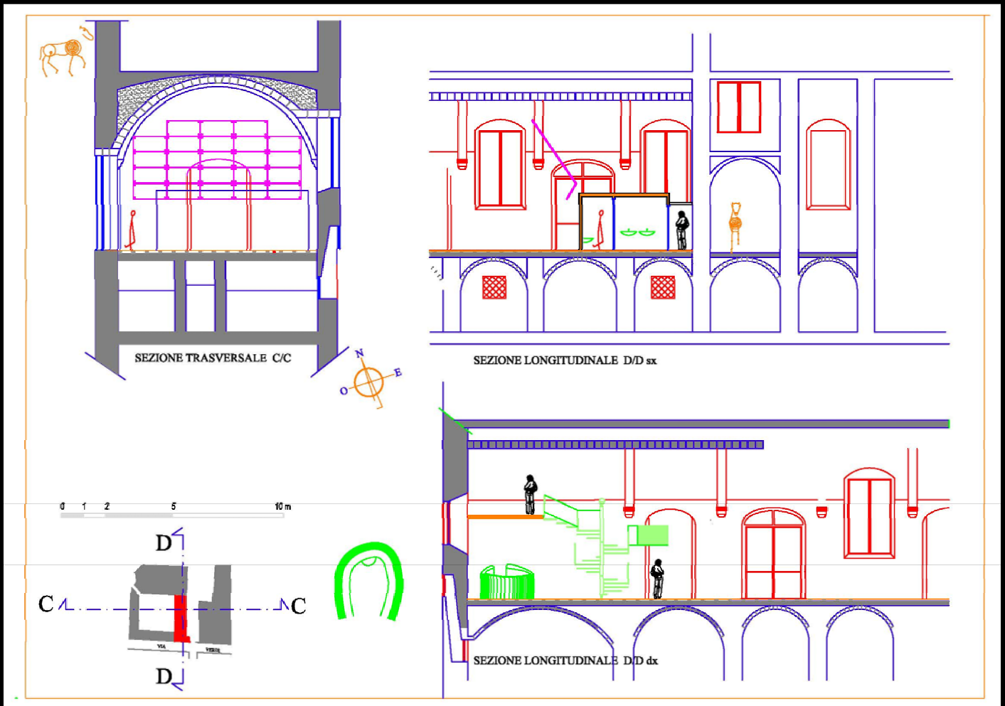
Sezione longitudinale
